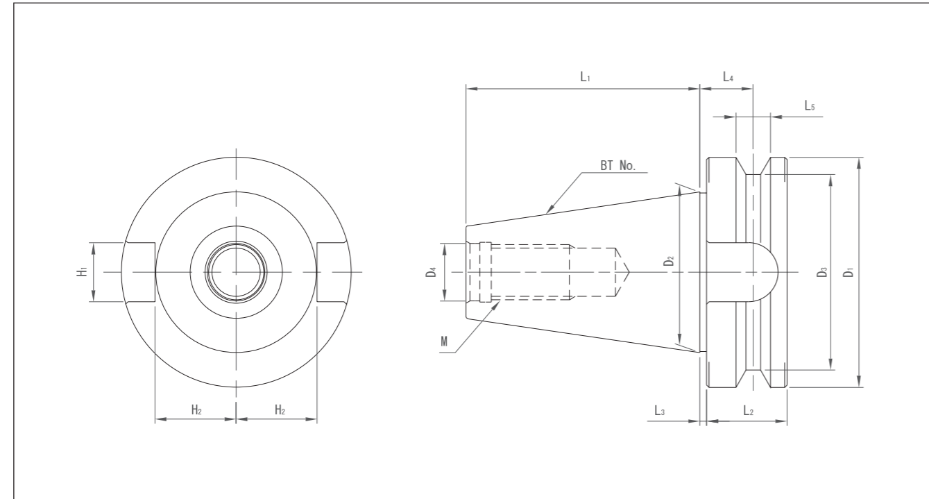
BT寸法表 BT Dimension Table
