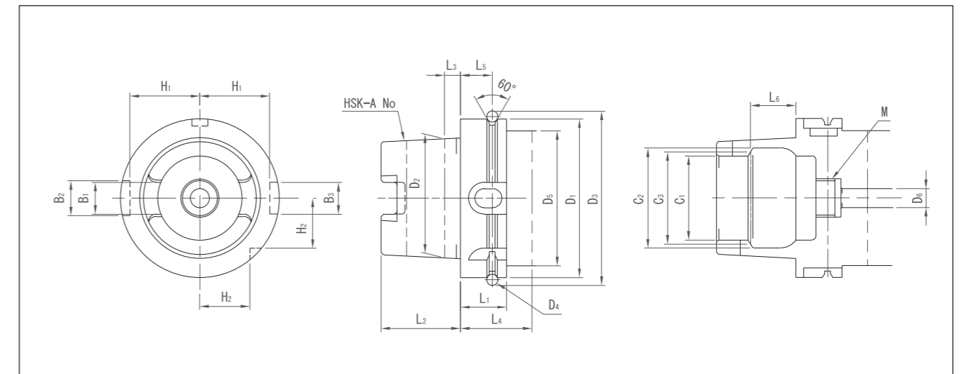
HSK寸法表 HSK Dimension Table
