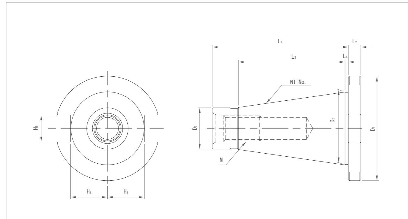
NT寸法表 NT Dimension Table
